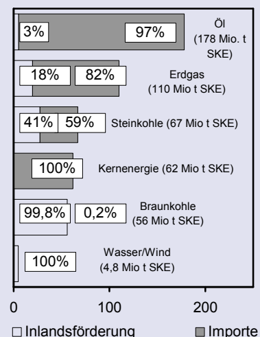
Energie-Importabhängigkeit Deutschland, 2003
