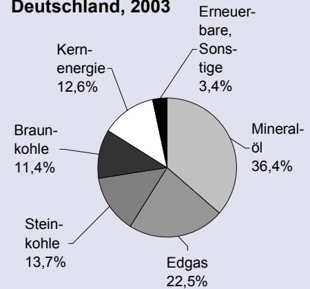
Primärenergieverbrauch Deutschland, 2003
